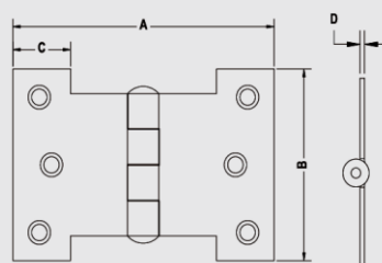
Dobradiça Palmela Linha 840
