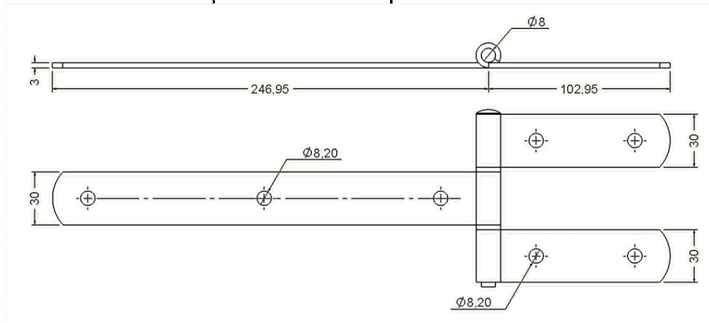
Desenho Técnico – Dobradiça 790 Haste Dupla Parafusar – 10”:
